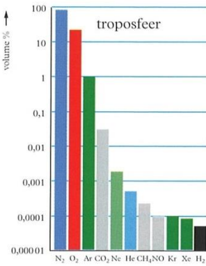
atmosfeer van de aarde
