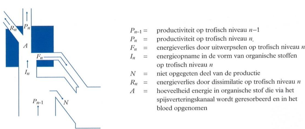
■ Energiestroom door trofische niveaus: assimilatie-efficiëntie ( A/I ) en productiviteitsefficiëntie ( P/A ) van een graslandmodel.
