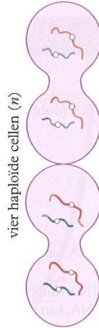
⑩ telofase II en cytokinese (n)
